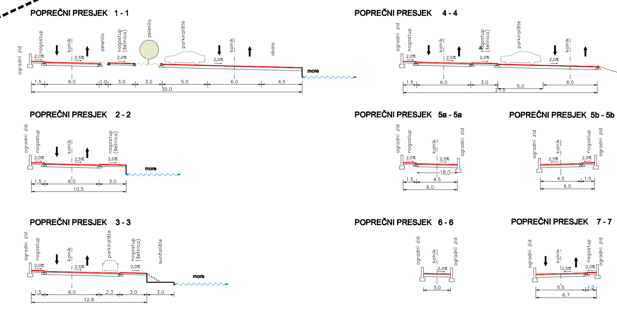
POPREČNI PRESJCI MJ. 1:250
